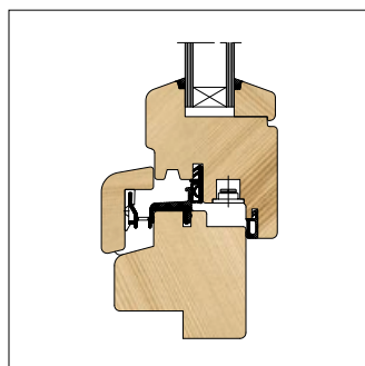
Voor naar binnendraaiende ramen
