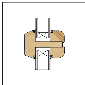
Kruisroeden glasdelend in diverse breedtes
