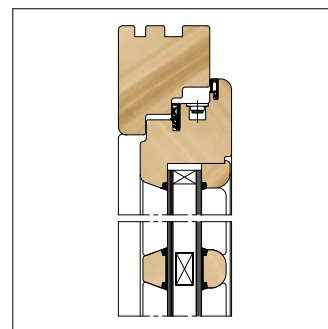
Kruisroeden aan twee zijden opgelijmd met afstandhouder tussen het glas, diverse breedtes mogelijk.
