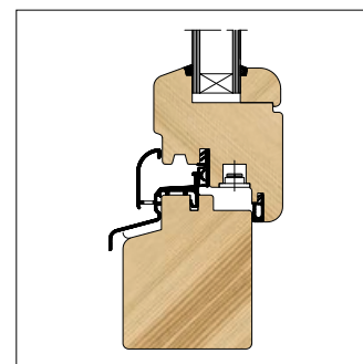
Ook leverbaar met afgeronde glaslat
