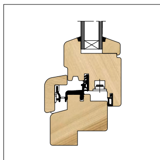
Voor naar buitendraaiende ramen
