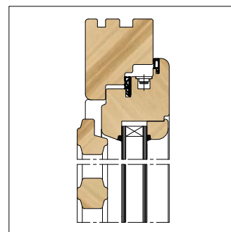
Voorzet kruisroeden aan de buitenzijde afneembaar
