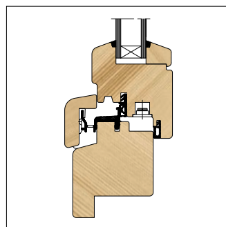
Met aanslag voor montage in een stelkozijn
