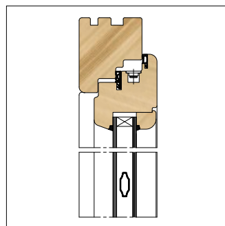
Kruisroeden tussen het dubbelglas
